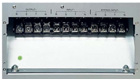
Block de terminales entrada/salida
